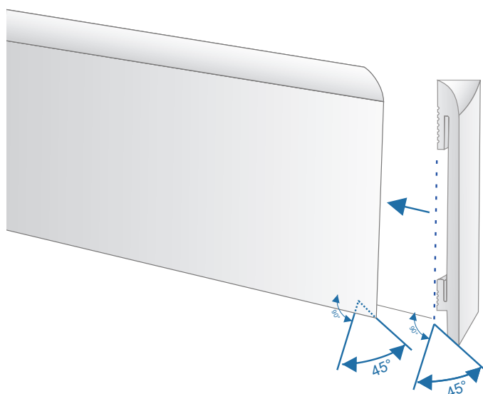
Tworzenie zakończenia bocznego listwy
